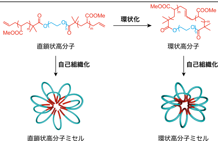
図 1 直鎖状高分子と環状高分子の分子構造とそれぞれから形成されるミセルの模式図。赤い部分が疎水部、水色の部分が親水部を示す。
